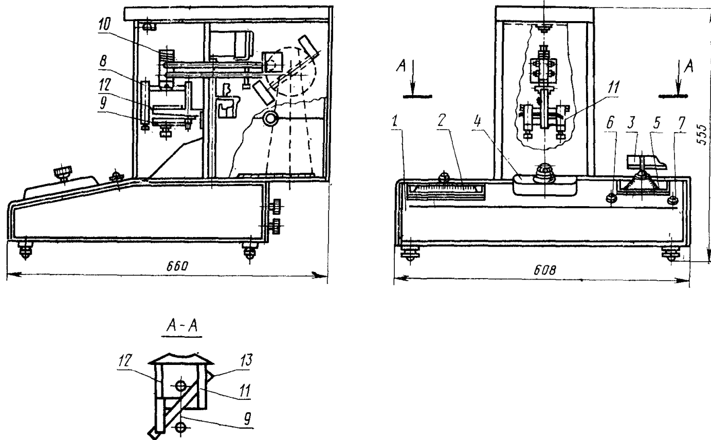
Схема прибора ППТ-4 для определения стойкости тканей и материалов к прожиганию
