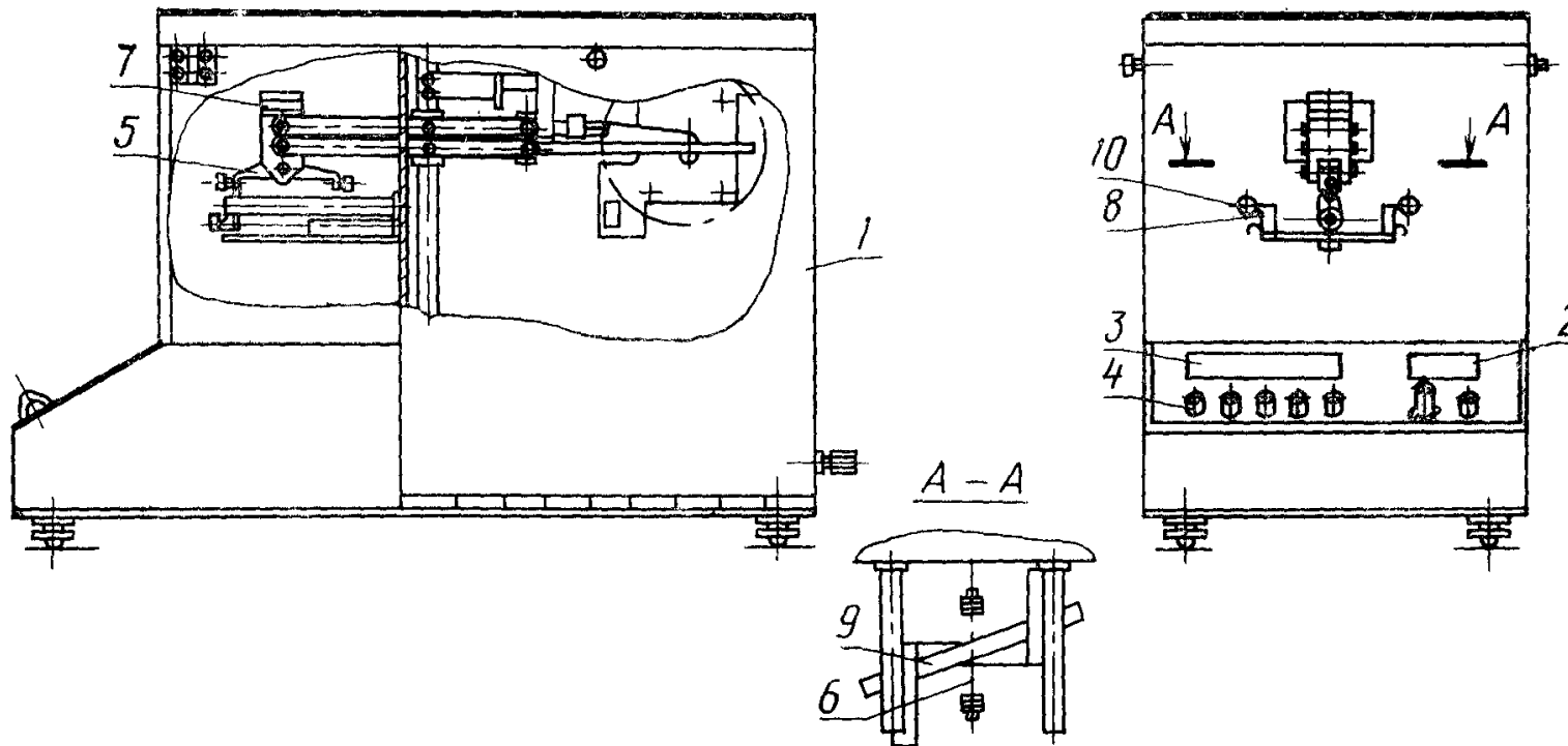
Схема прибора типа ППТ для определения стойкости тканей и материалов к прожиганию
