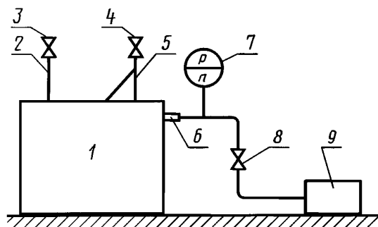
1 — резервуар; 2 — всасывающий трубопровод; 3, 4 — запорные краны; 5 — нагнетающий трубопровод; 6 — уровнемер; 7 — манометр; 8 — пус- ковой кран; 9 — компрессор
