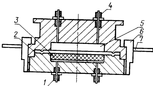
Диффузионная ячейка (газохроматографический метод)
