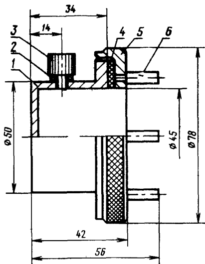
Диффузионная ячейка (гравиметрический метод)
