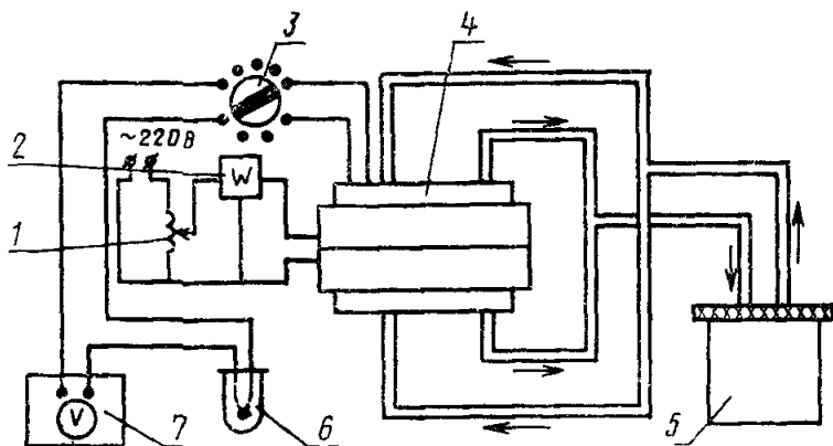
1—автотрансформатор, 2—ваттметр, 3—переключатель термомпар 4—рабочая часть 5—термостат 6—холодный спай термопар 7—электронно цифровой вольтметр
