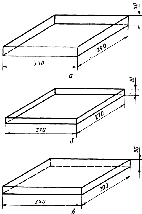
а—поддон; б—прижимная рамка; в—крышка
