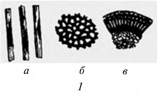
1 — ржавчина льна на мертвом соре в семенах: a — пятна зимней стадии на обломках веточек; б — вид под микроскопом коростинки зимней стадии ржавчины льна; в — зимние споры ржавчины льна; 2 — фузариоз льна: a — на семенах льна; б — конидии гриба; 3 — антракноз льна: a — на семенах льна; б — спороношение гриба; 4 — крапчатость льна: a — на семенах льна; б — мицелий гриба; 5 — бактериоз льна: a — на семенах льна; б — бактерии и их споры; 6 — аскохита льна: a — колония на агаре; б — пикнида аскохиты с выходящими спорами; 7 — полиспороз льна: a — колония на агаре; б — конидии полиспоры
