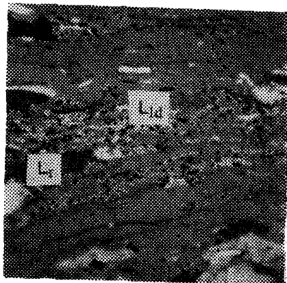
Отраженный свет Масляная иммерсия 400× L ld — липтодетринит L r — резинит Черт. 10
