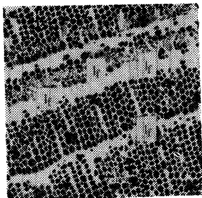
Отраженный свет 100 \times I f — фузинит Черт. 8
