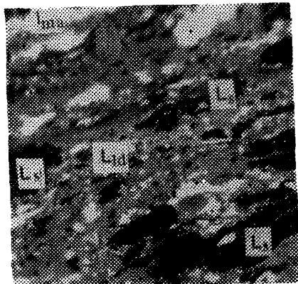
Отраженный свет Масляная иммерсия 400× L s — споринит I ma — макринит L ld — липтодетринит Черт. 9
