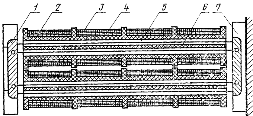
1—ядро; 2—каркас соленоида; 3—намагничивающая обмотка; 4—измерительная обмотка; 5—испытываемые листы; 6—изоляционная прокладка; 7—держатель ярма
