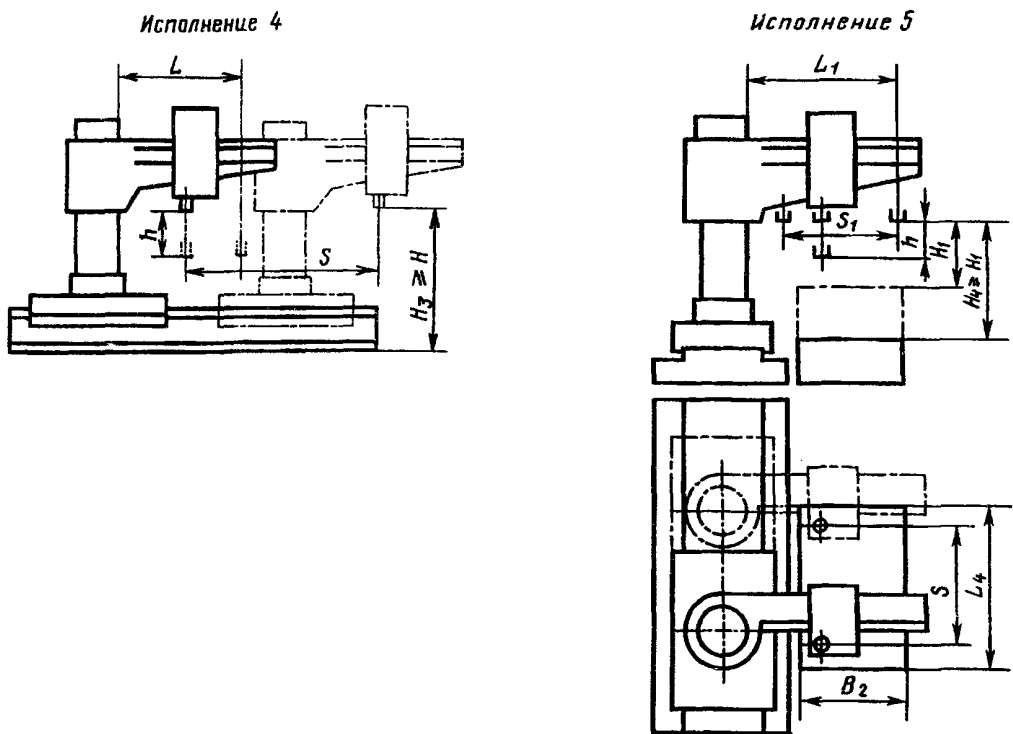
Размеры, мм
