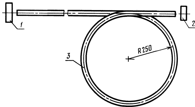
1 — привод; 2 — спидометр; 3 — гибкий вал
