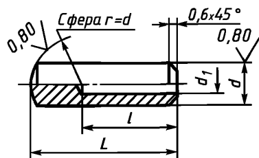
Исполнение 1
