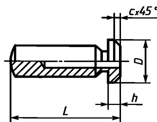
Исполнение 2
