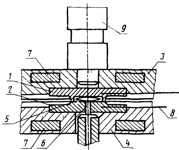
Испытательная камера
