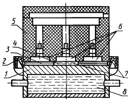
Схема электродного устройства
