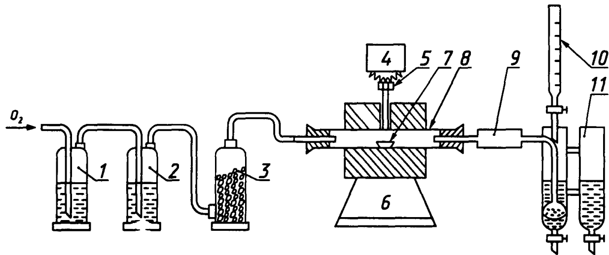
1—2 — барботеры для очистки кислорода; 3 — осушительная колонка; 4 — потенциометр; 5 — термопара; 6 — трубчатая печь; 7 — фарфоровая неглазурованная лодочка; 8 — фарфоровая неглазурованная трубка; 9 — пылеуловитель; 10 — микробюретка; 11 — абсорбционный аппарат
