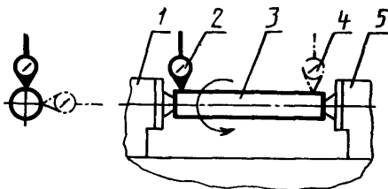
Черт 4
