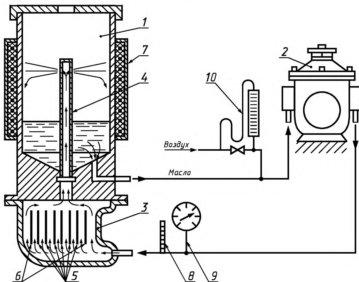
Схема установки ПЗЗ
