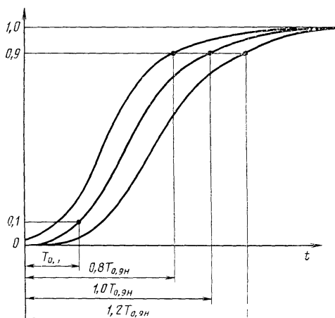
ГРАФИК ПЕРЕХОДНОГО ПРОЦЕССА
