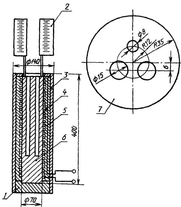
1 — огнеупорный материал; 2 — зеркало; 3 — асбестоцемент; 4 — слюда; 5 — смесь магнез и асбеста; 6 — алюминиевая бронза; 7 — положение отверстий
