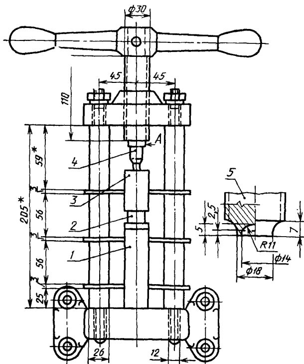
1 — трубка направляющего устройства; 2 — форма; 3 — направляющее устройство; 4 — выталкивающий поршень; 5 — конец винта А
