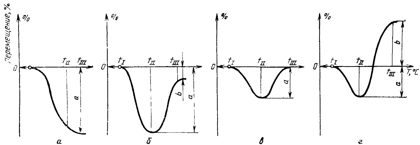
Рисунок 1 — Кривые дилатации
