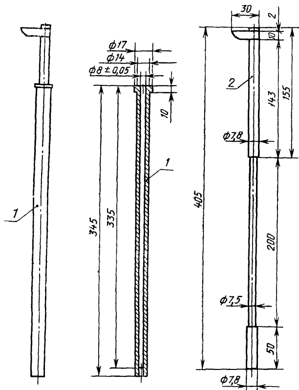
Рисунок 5 — Дилатометрическая трубка и поршень
