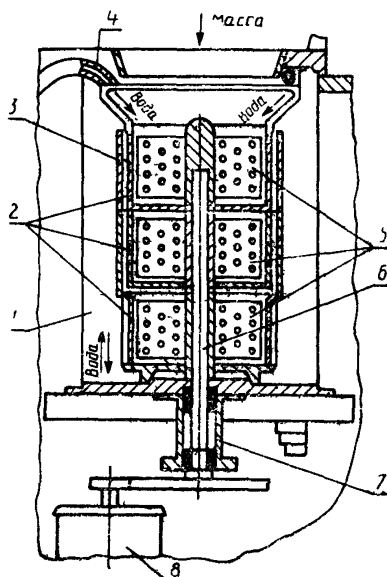
1 — резервуар; 2 — корпус сетки; 3 — втулка дистанционная; 4 — спрыск; 5 — лопастные мешалки; 6 — вал; 7 — привод; 8 — электродвигатель
