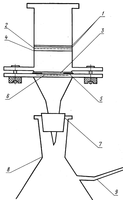
Модифицированный прибор Зейтца
