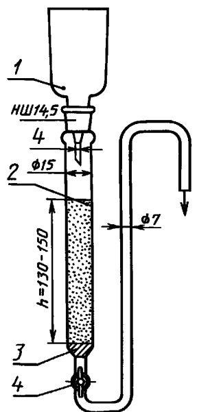
1 — резервуар вместимостью 50 см 3 ; 2 — колонка с кадмием; 3 — стекловата; 4 — кран
