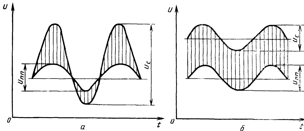
Осциллограмма скорректированного КС с переходной помехой на модулирующих частотах
