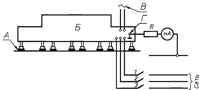
А — подставка из изоляционного материала; Б — посудомоечная машина; В — питание цепей управления; Г — болт заземления; 1, 2, 3 — однополюсные выключатели; мА — миллиамперметр класса 1,0; R — резистор
