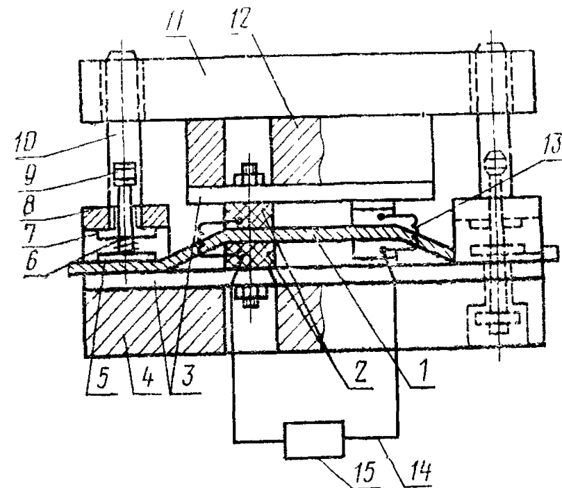
Электродное устройство
