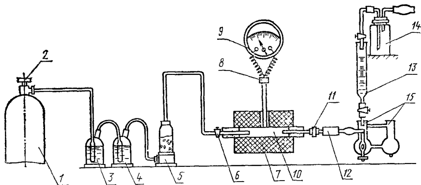
1 — баллон с кислородом, 2 — редукционный вентиль, 3, 4 — склянки для очистки кислорода, 5 — колонка для осушения кислорода, 6 — треххвостовой крап, 7 — трубчатая печь, 8 — платино платинородиевая термопара, 9 — гальванометр, 10 — фарфоровая неглазурованная трубка, 11 — зажим, 12 — пылеуловитель, 13 — бюретки, 14 — склянки, 15 — абсорбционный аппарат
