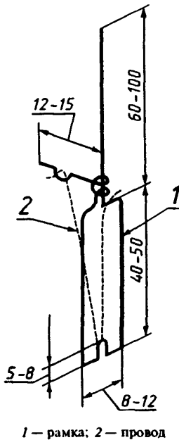
1 — рамка; 2 — провод
