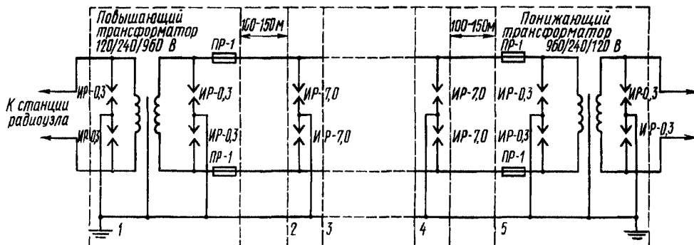
1 — выводная опора; 2, 4 — опоры; 3 — воздушная стоечная или столбовая линия; 5 — оконечная опора
