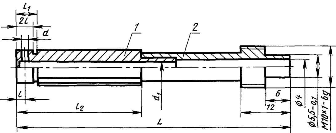
1—вставка; 2—переходник Черт. 8
