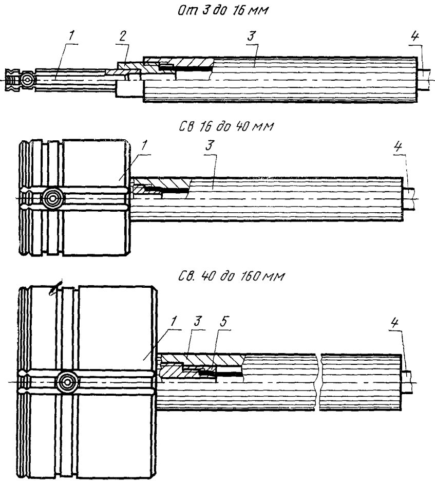
1—вставка; 2—переходник; 3—ручка; 4 —шланг, 5—гайка
