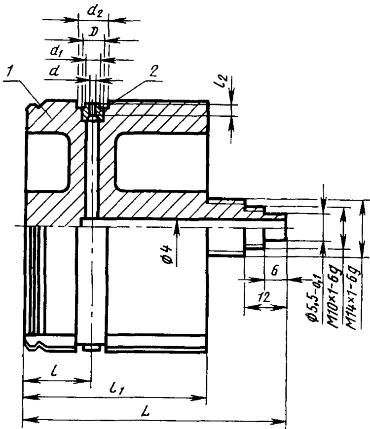
1—вставка; 2—вставное сопло Черт. 6
