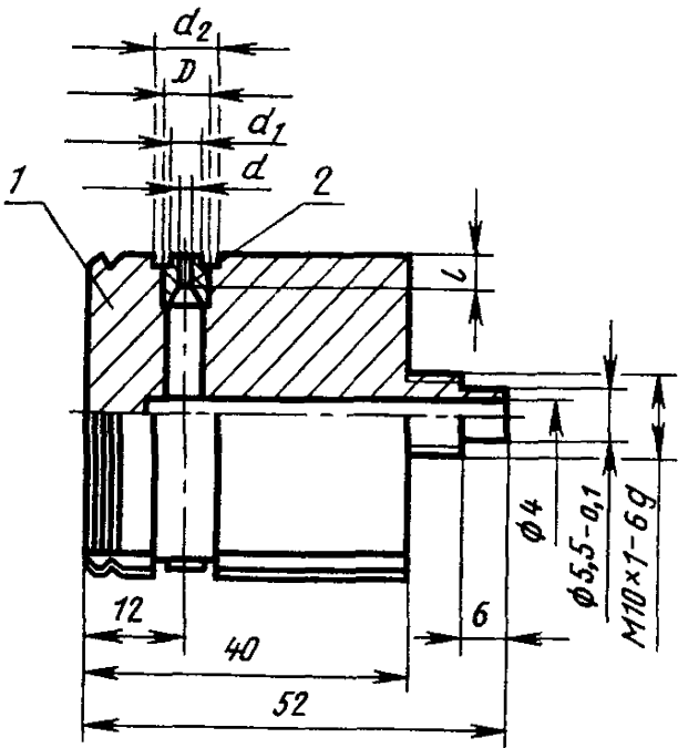
1—вставка; 2—вставное сопло Черт. 5
