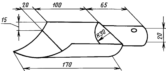
Щуп для отбора точечных проб
