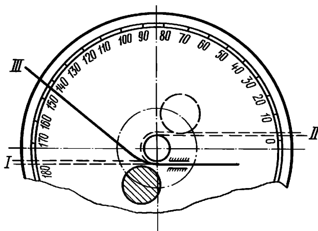
Схема испытания ленты на пружинность
