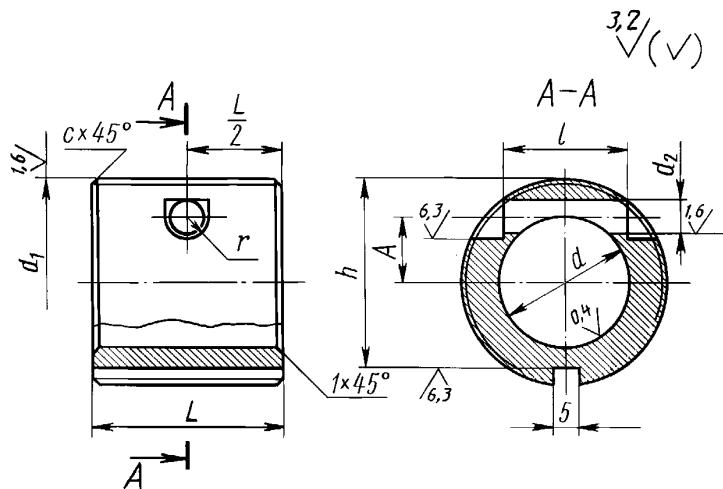
Черт. 2 Размеры в мм
