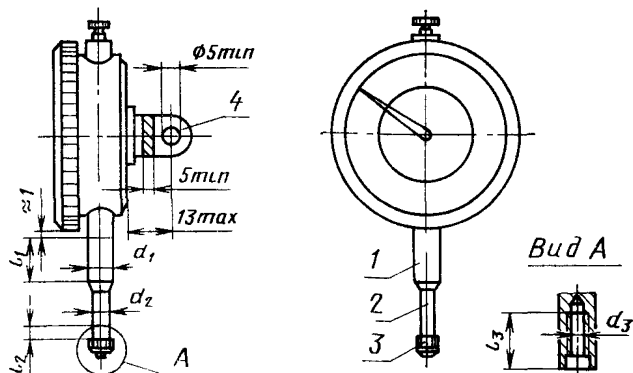
1 — присоединительная гильза, 2 — измерительный шток, 3 — измерительный наконечник, 4 — ушко
