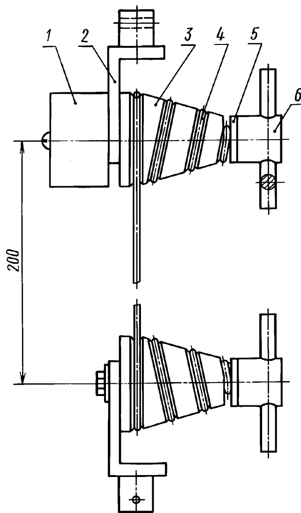
1 — противовес; 2 — корпус; 3 — улитка; 4 — образец провода; 5 — шайба; 6 — зажим
