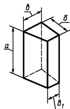
Рисунок 6 — Электродный кирпич
