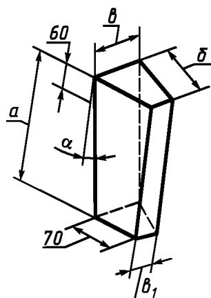
Рисунок 7 — Внешний электродный кирпич
