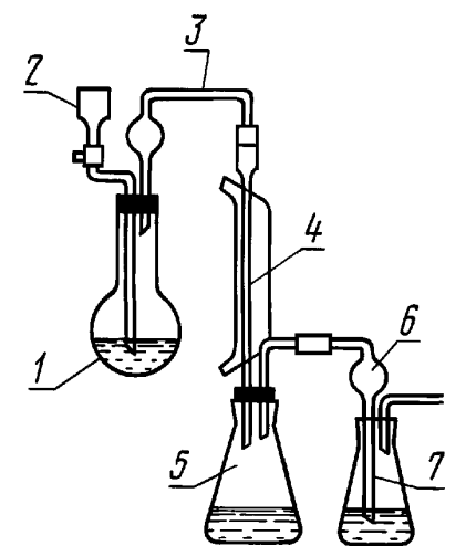
Установка для отгонки мышьяка
