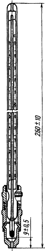
Термометр с гильзой и чашечкой
