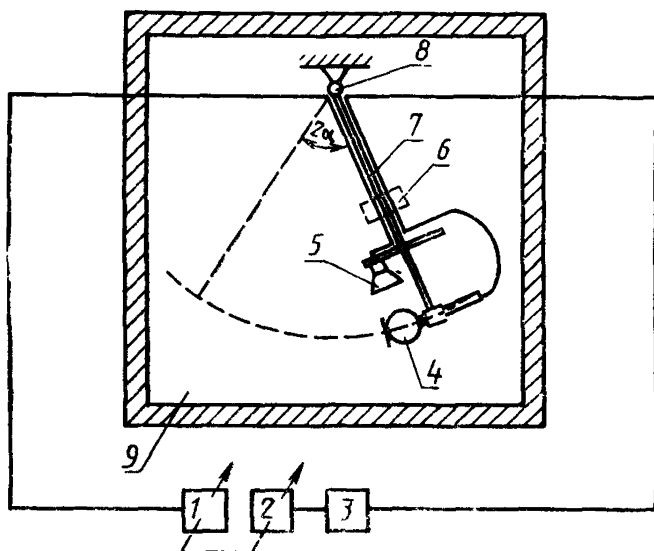
1 — низкочастотный генератор сигналов (п 121), 2 — анализатор спектра (п 15) 3 — самописец уровня (п 12), 4 — испытуемый микрофон, 5 — излучатель (п 112), 6 — инерционная масса, 7 — кронштейн, 8 — горизонтальная ось, 9 — звукомерная заглушенная камера (п 118)
