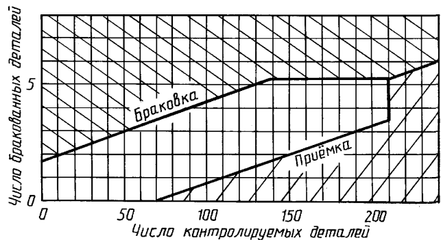
Диаграмма Вальда
