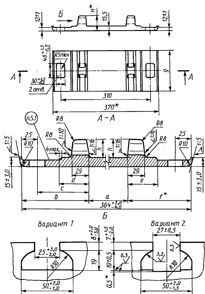
Подкладка типа КБ
