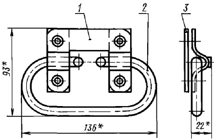
Ручка 1 ОКП 72898 84301
