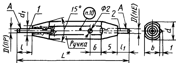
Калибр-пробка двусторонний
