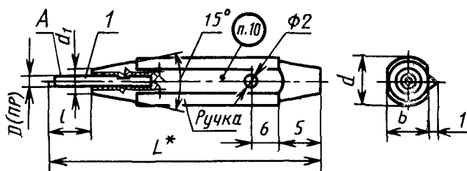
Калибр-пробка односторонний
