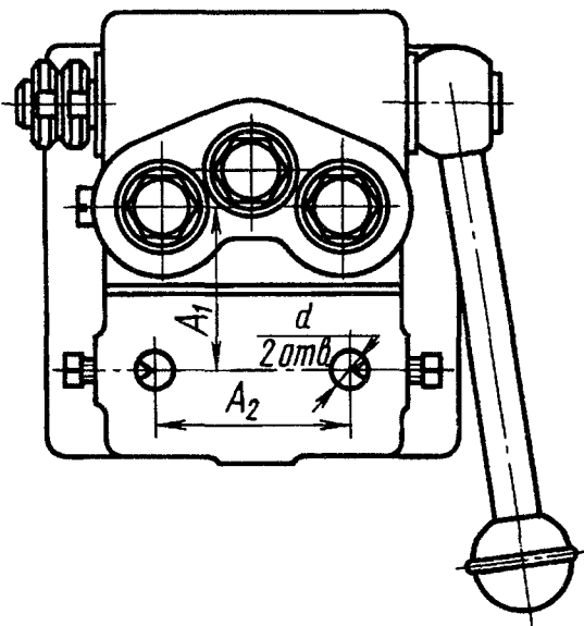
Исполнение 2 Вид сверху Плита (поз. 2) не показана
