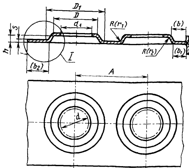
Отбортовка типа 3
