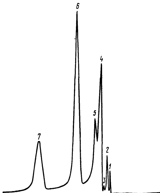
Типовая хроматограмма технической муравьиной кислоты
