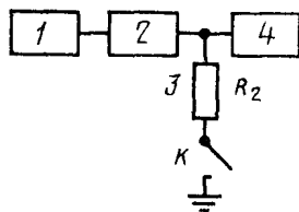
1—генератор 2—испыта- емый фильтр 3—дополни- тельное сопротивление R_2 4—вольтметр К—выключа- тель
