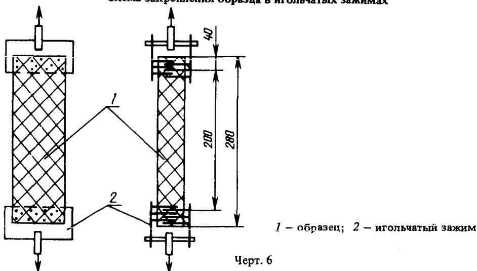
Схема закрепления образца в игольчатых зажимах
