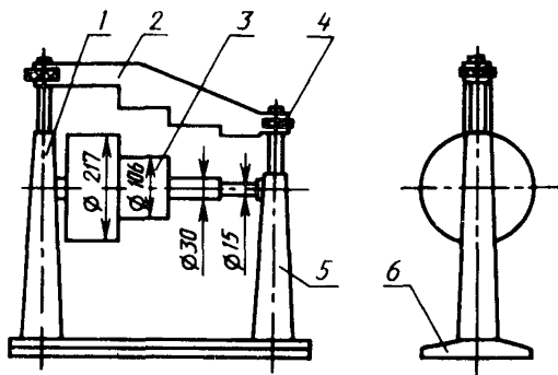
1 — опора; 2 — прижимная планка; 3 — валик; 4 — гайка; 5 — опора; 6 — основание
