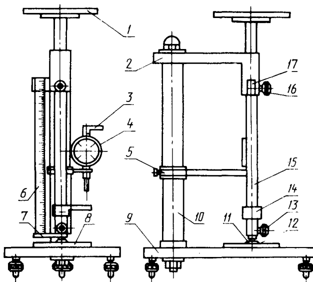
Прибор для определения сжимаемости
