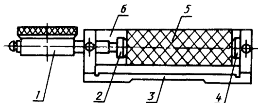
Устройство для определения линейной усадки
