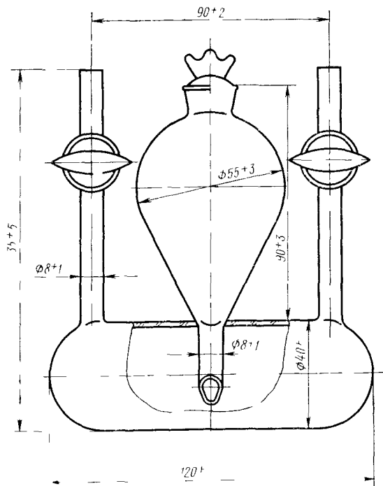
Испаритель
