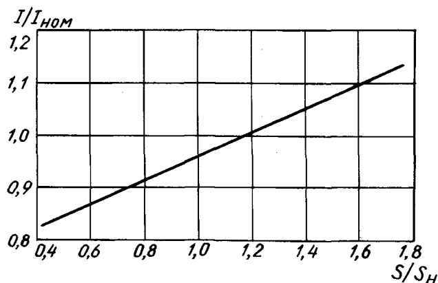
Зависимость тока предохранителя от сечения кабеля
