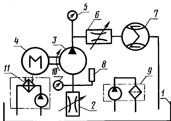
Принципиальная схема испытательного стенда
