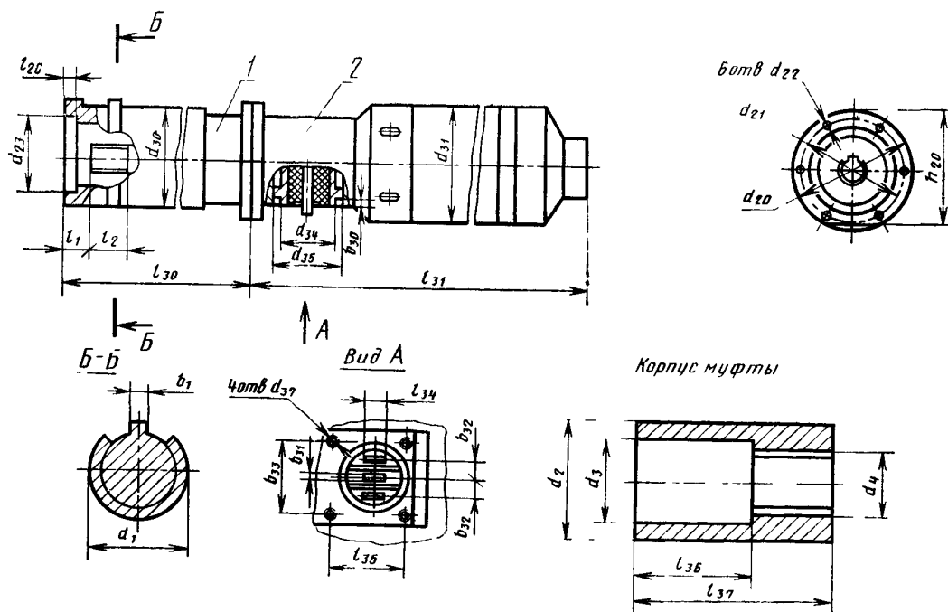
1—протектор, 2—электродвигатель
