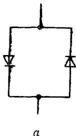
Ограничитель напряжения на уровне \pm(0,5—0,6) В
