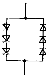
Ограничитель напряжения на уровне \pm(1,5—1,8) В
